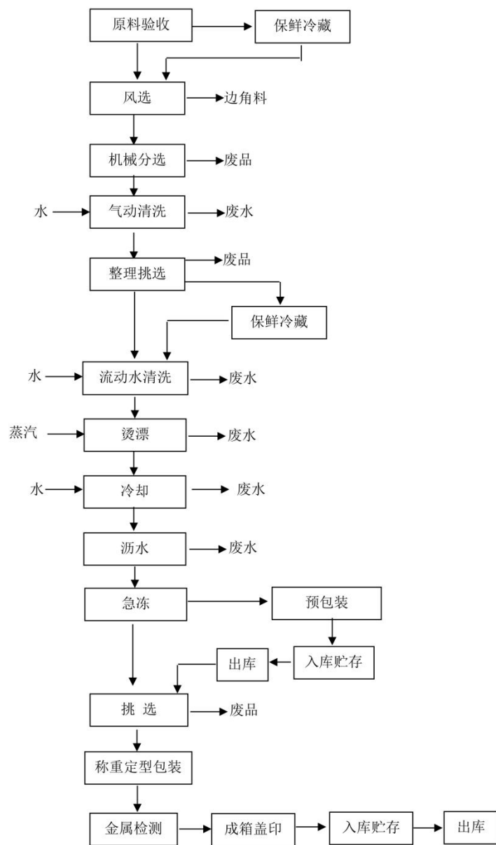
图 3 生产工艺流程图
